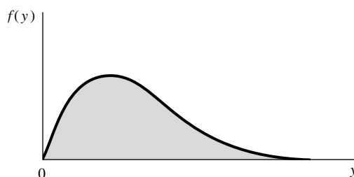
FIGURA 4.15 Función de densidad de probabilidad sesgada
