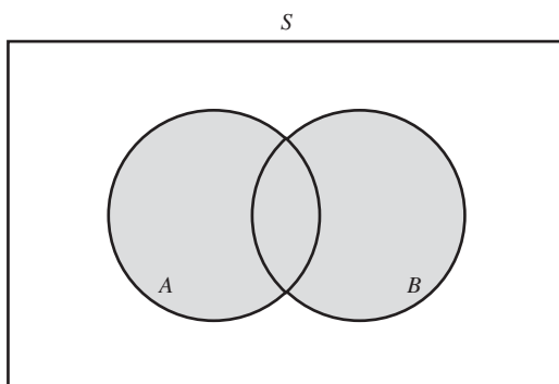
FIGURA 2.3 Diagrama de Venn para A \cup B
