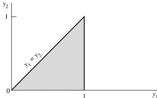
FIGURA 5.7 Región sobre la cual f(y_1, y_2) es positiva, Ejemplo 5.12
