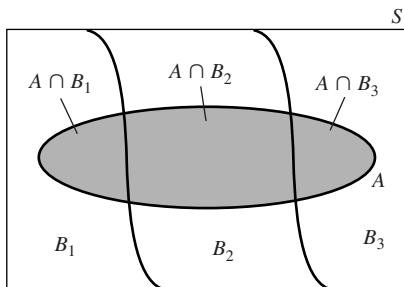
FIGURA 2.12 Descomposición del evento A
