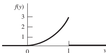
FIGURA 4.6 Función de densidad para el Ejemplo 4.3
