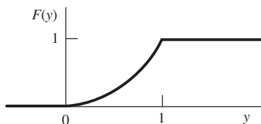
FIGURA 4.7 Función de distribución para el Ejemplo 4.3
