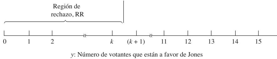
FIGURA 10.1 Región de rechazo, RR = \{y \leq k\} , para una prueba de la hipótesis H_0: p = .5 contra la alternativa H_a: p < .5
