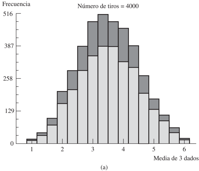
FIGURA 7.1 (a) Distribución de muestreo simulado para \bar{Y} , Ejemplo 7.1; (b) media y desviación estándar de los 4000 valores simulados de \bar{Y}
