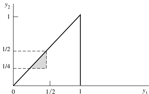
FIGURA 5.5 Región de integración para el Ejemplo 5.4
